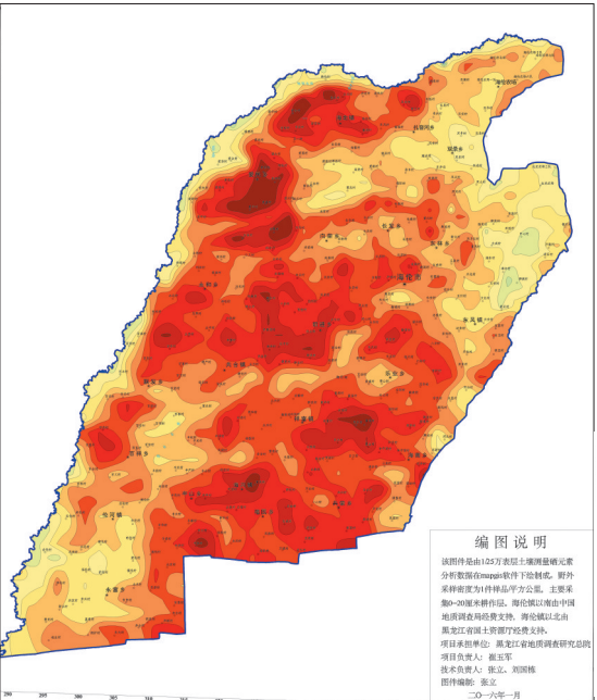
海伦市 1/25 万表层土壤地球化学测量硒元素地球化学图
