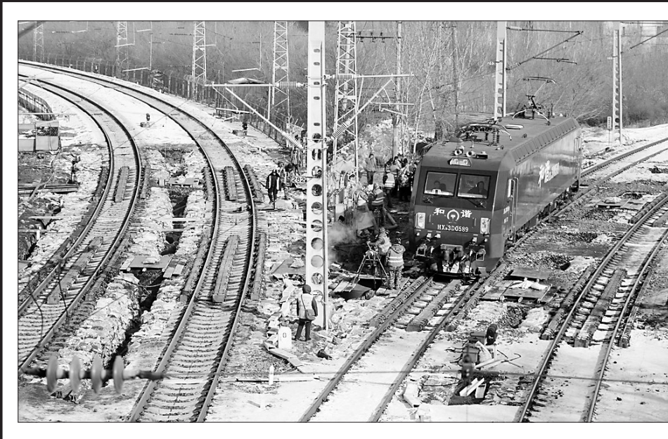
日前,哈尔滨市彩虹桥附近的铁路上正在进行一面街打通工程,该工程北起一面街,南至月牙街,双向六车道,预计六月份可完工,届时南岗区的车辆可以从地道驶入道里区。图为工人们正在对铁轨加固,并打桩。 本报记者 苏强摄
