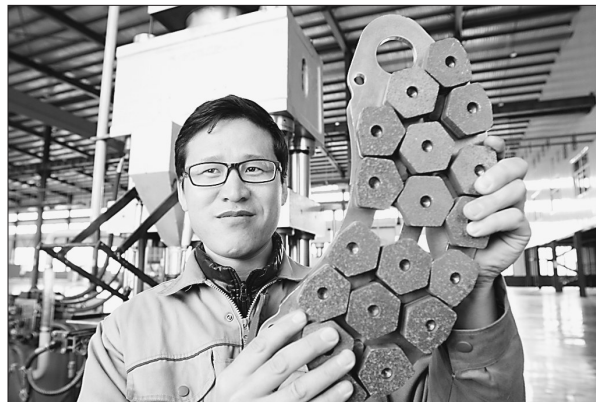
杜尔伯特蒙古族自治县工业园区的瑞瑞摩擦材料公司,生产橡胶、动车、货运列车、地铁等的制动片。企业拥有粉末冶金、合成材料两条生产线,年加工粉末冶金摩擦材料和有机合成摩擦材料等多种摩擦材料体系制品1000万片。图为工人展示高铁列车片。孟立威 本报记者 李飞 苏强摄
