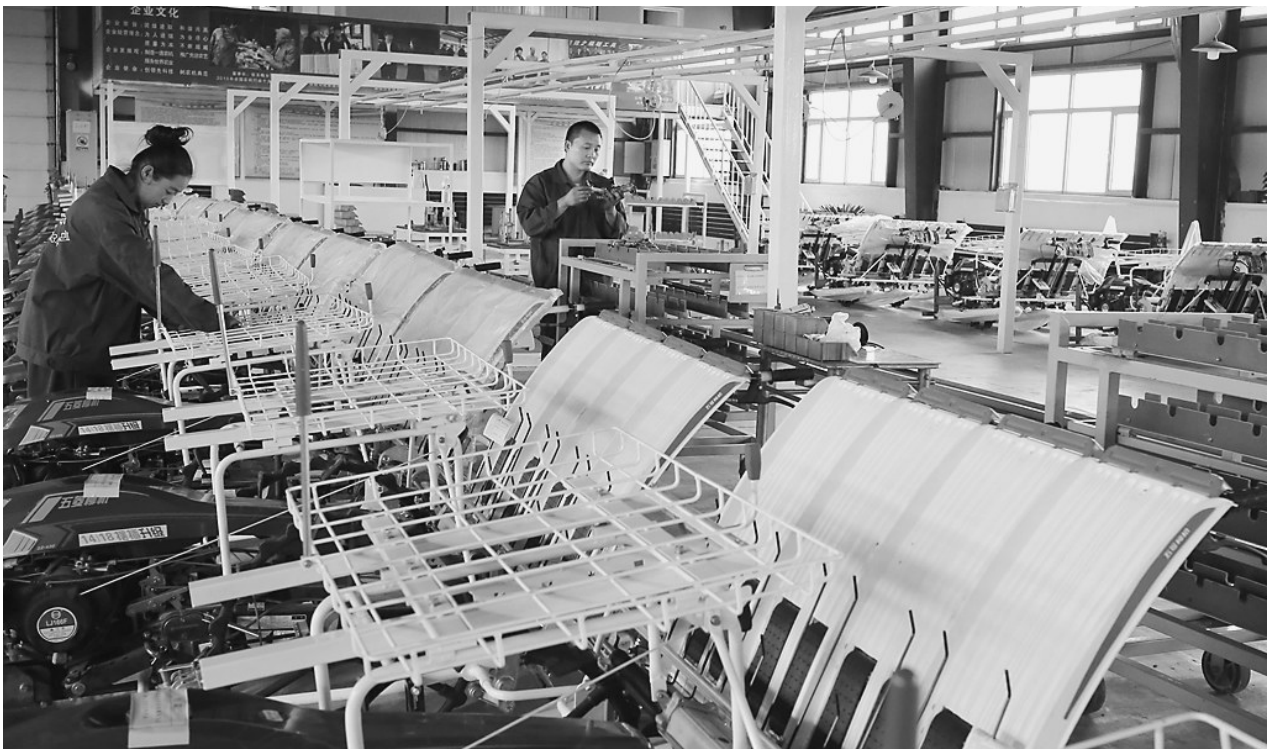
日前,铁力经济开发区玉梅农机装备有限公司的车间里,一派忙碌的景象,一排排水稻插秧机走下生产线,300多台插秧机准备发往吉林、辽宁等地。图为技术人员正在给水稻插秧机做最后的调试。
