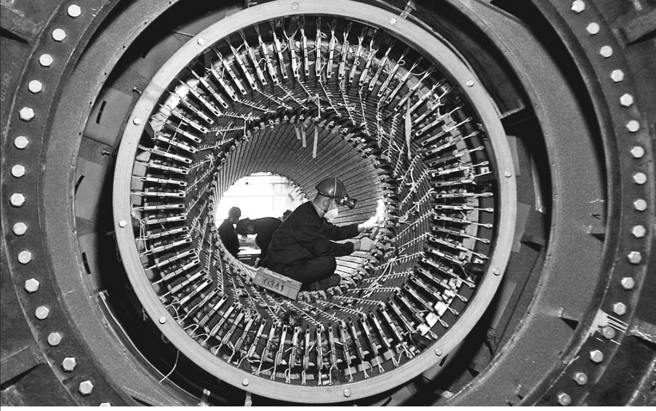
哈电集团哈尔滨电机厂有限责任公司积极开发节能环保产品。公司技术人员在生产天津津粮城项目燃气轮发电机产品过程中,对定子线圈进行了国产化研制并取得成功,性能指标优于国外产品,推动了我国燃气轮发电机制造技术的发展。
