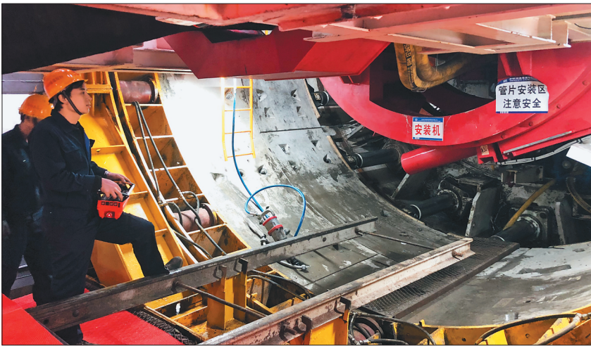
“松江1号”盾构机施工现场。
