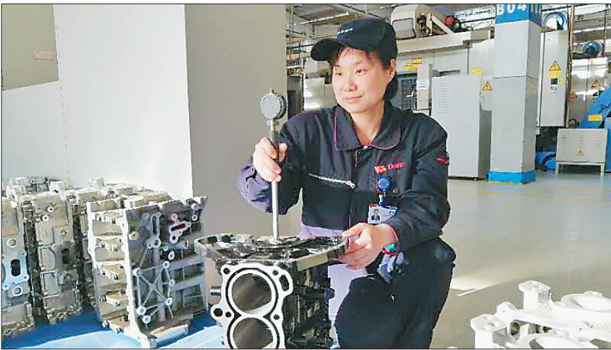
苗秀正在测量516K缸体主轴承孔孔径。
