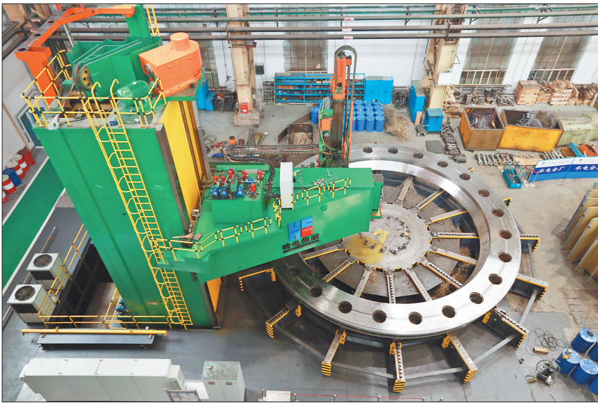
哈电集团电机公司16米立车加工白鹤滩4号底环。
