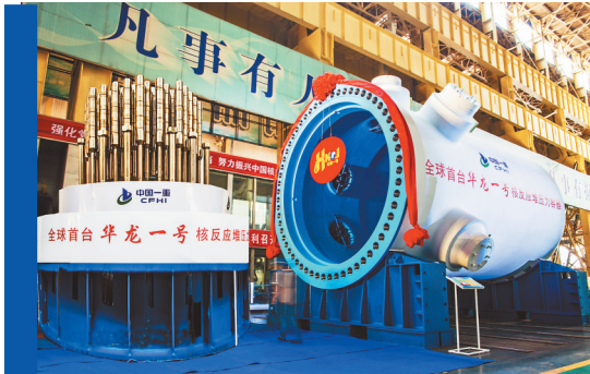
中国一重全球首台“华龙一号”核反应堆压力容器发运。
