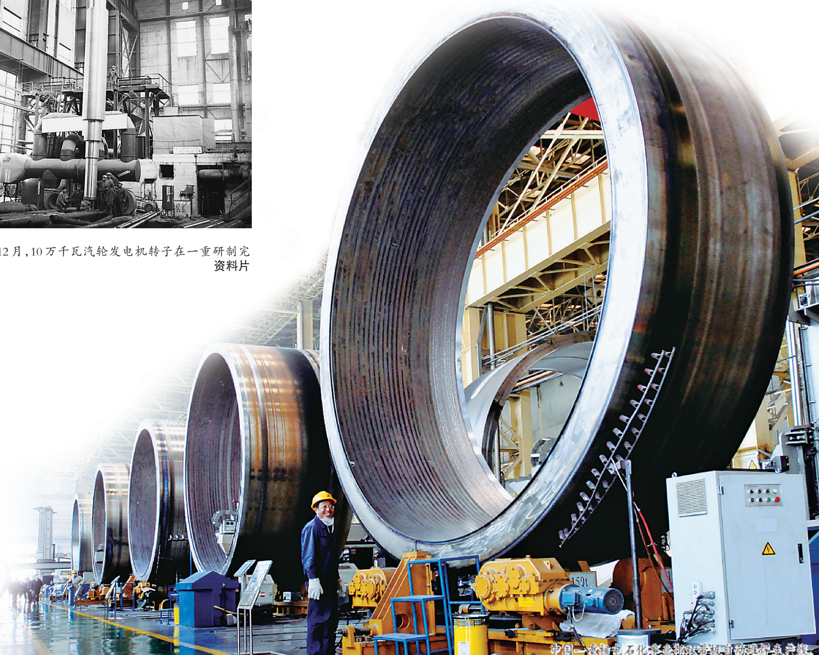
中国一重造石化工业用大型汽轮机转子
