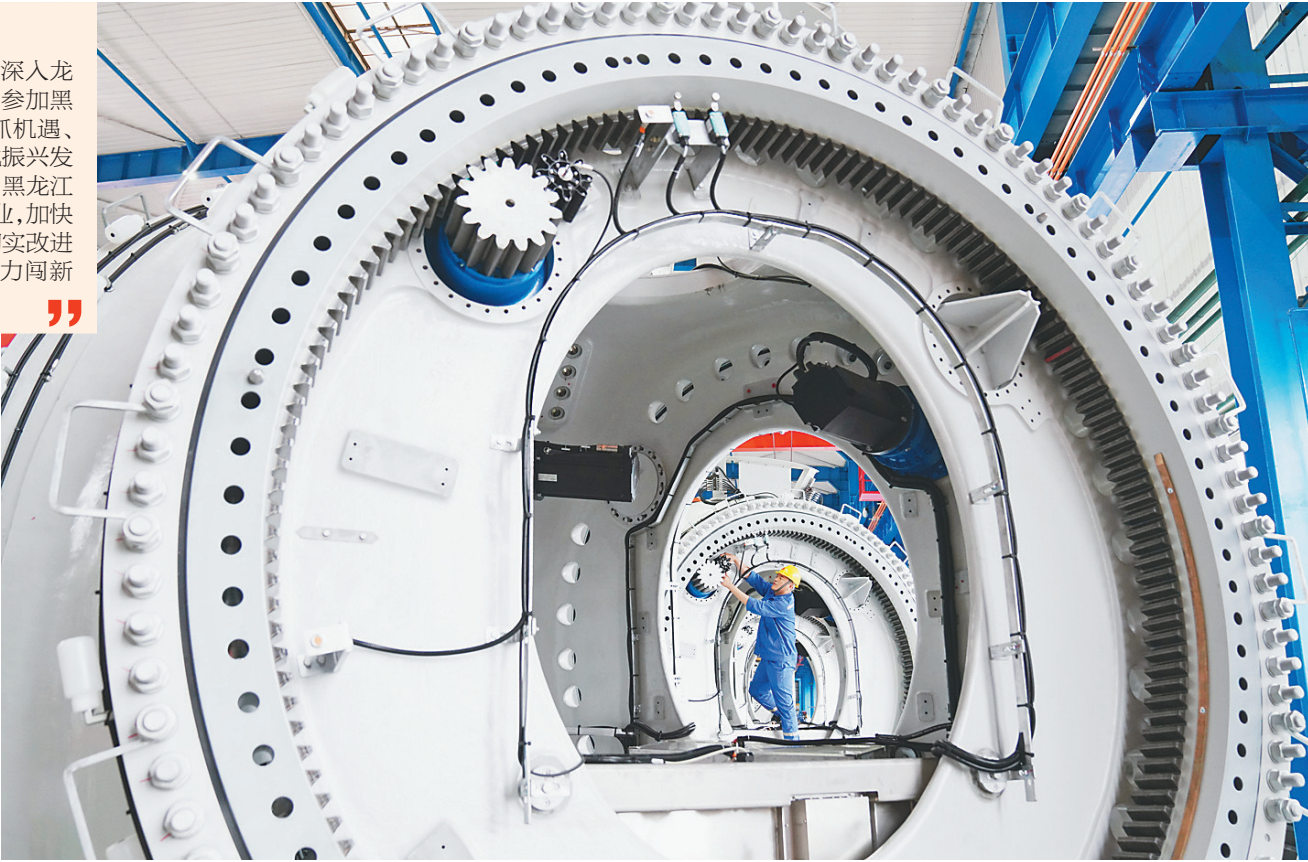
在齐齐哈尔市中国一重集团有限公司风电装备生产制造厂生产车间,工人进行生产作业(2021年7月1日摄)。
