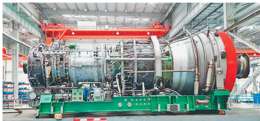
第七〇三研究所牵头研制的我国首台套30MW级燃气轮机驱动压缩机。 图片由受访单位提供
