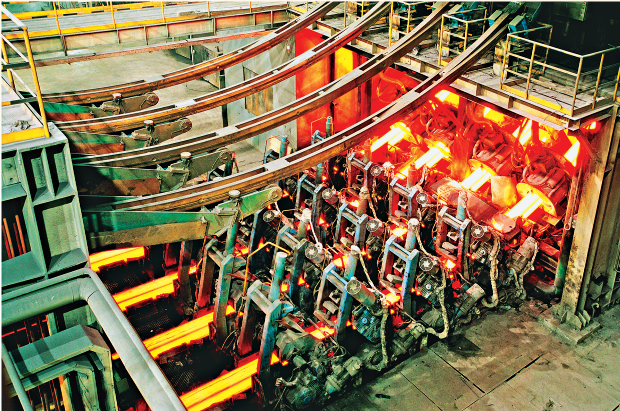
建龙北满特钢四机四流大方坯生产线正在全力生产。
