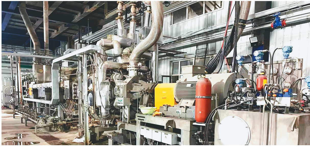
粉料造粒机组。
