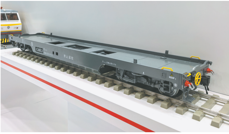
中车齐车公司展出的时速160公里快捷平车模型。
