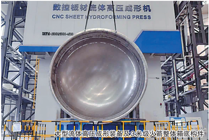
大型流体高压成形装备及3米级火箭整体箱底构件
